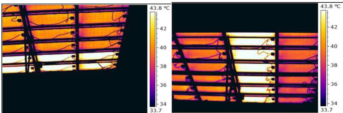
Obr. 38 Chybné zapojení fotovoltaického panelů [2]
