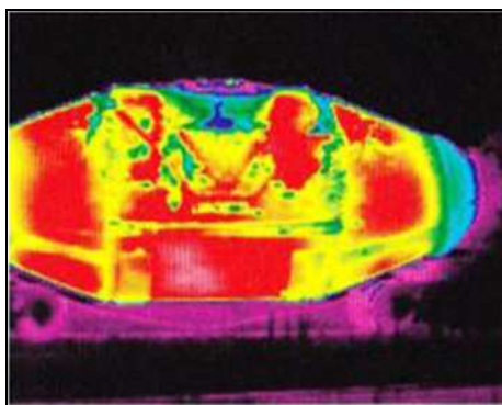
Obr. 21 Směrnicevá termografie – Dopravní vozík naplněný roztaveným kovem [5]
