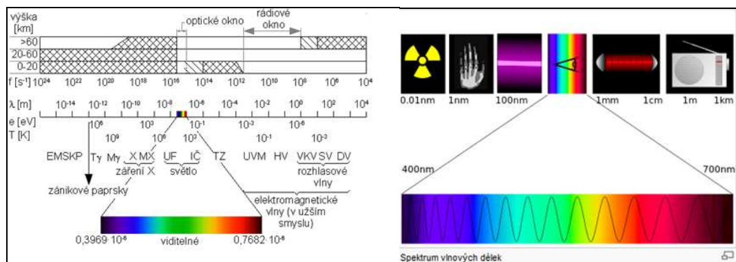
Obr. 9 Elektromagnetické spektrum [6]
