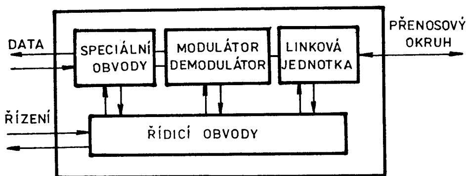
Blokové schéma modemu
