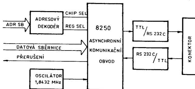
Schéma zapojení obvodů rozhraní RS 232 C a blokové schéma adaptéru
